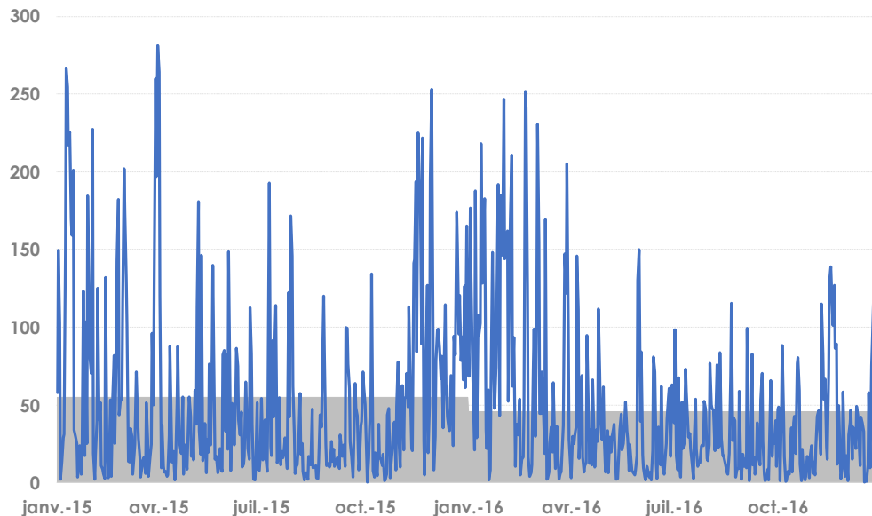
Profil de production journalière d'un par éolien (MWh)
