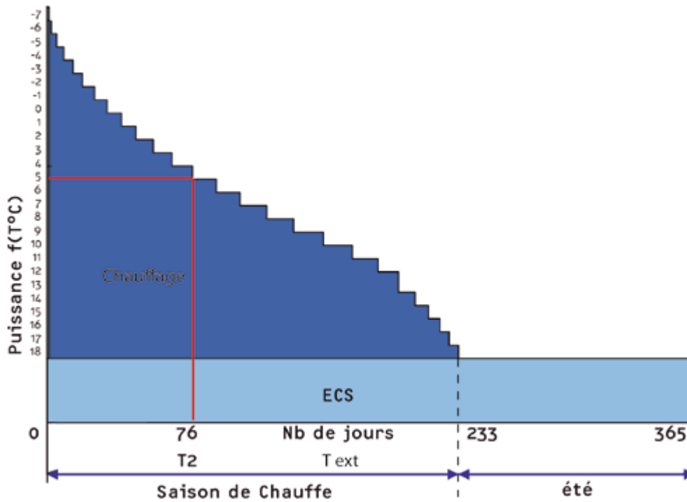
Courbe monotone de charge (Chauffage et ECS) avec une T_{\text{eb}} = -7^{\circ}\text{C}
